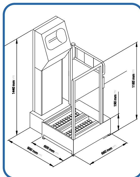
DETTAGLIO 04:
